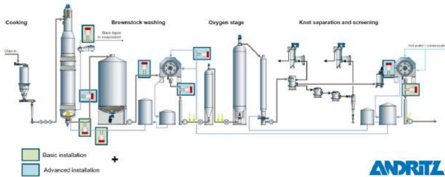
KUVA 7. Advanced-ratkaisu pesulinjan toiminnan mittaamiseen perustuen online-refraktometreihin (kuva Andritz).
