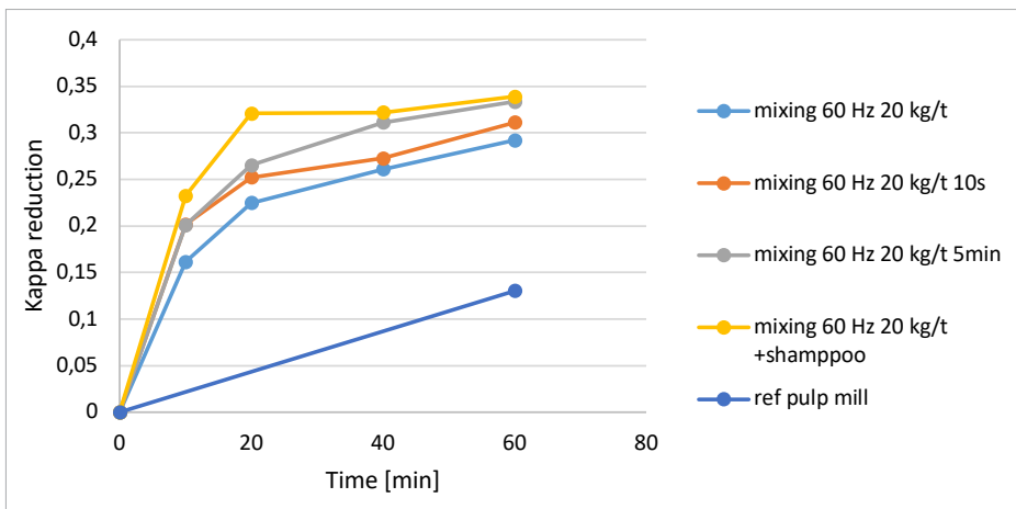
KUVA 5. Sekoituksen ja dispergointiaineen käytön vaikutus kappareduktioon. Sekoitussnopeus 2400 \text{ rpm}^{-1} , lämpötila 90 astetta, paine 7 baaria. (kuva Antti Pappinen)
