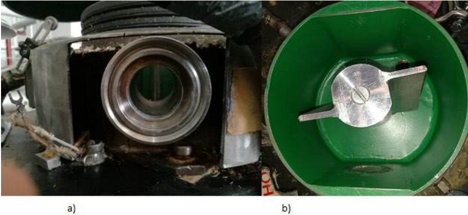
KUVA 1. Mark IV -laboratoriosekoittimen reaktorin kylkien tasaisille pinnoille on asennettu kaksi Sandvikin L-tyypin laippakiinnityksellä olevaa yhdettä, joiden kautta reaktoriin voidaan liittää mittausjärjestelmiä ja saada tarkempaa informaatiota reaaliaikaisesti. Kuvassa 1a Sandvikin L-tyypin laippa ja kuvassa 1b reaktori kuvattuna ylhäältä. (kuva Antti Pappinen)
