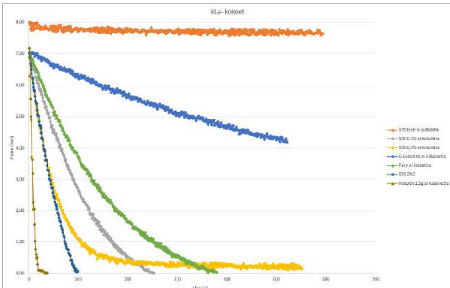
KUVA 3. Hapen aineensiirtokokeiden tulokset eri lisäaineilla (kuva Antti Pappinen).
