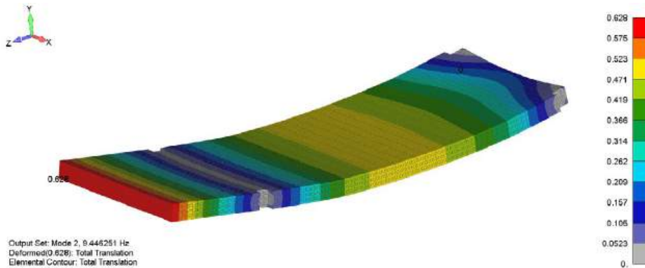
KUVA 9. Alinta ominaistajuutta (9,4 Hz) vastaava ominaismuoto, laatan symmetrinen puoliallotaivutus (kuva Stressfield Oy).
