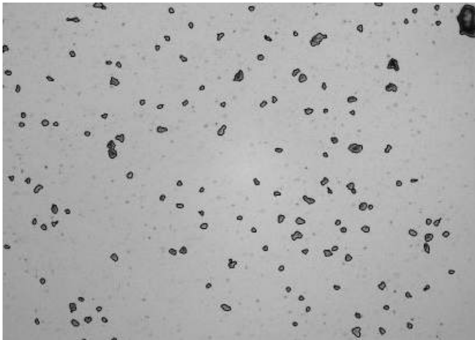
KUVA 3. Valmet Automationsin kameran ottama kuva flokkivedestä, josta analyysiohjelma on tunnistanut flokit ja ympyröinyt ne (kuva Yrjö Hiltunen).
