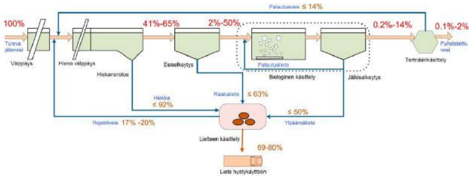
KUVA 1. Arvio mikromuovin kulkeutumisesta jätevedenpuhdistusprosessissa (mukailen Sun ym. 2019).
