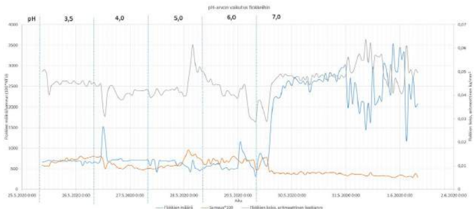
KUVA 4. pH-arvon muutoksien vaikutus flokkeihin.
