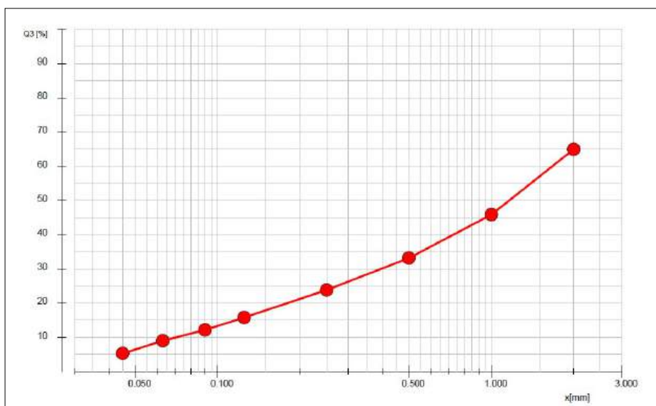
KUVA 3. Seulakoneella seulotun tiilen läpäisyprosentit käytetyille sihdeille. Seulotulle tielle tehty partikkelikokoanalyysit.
